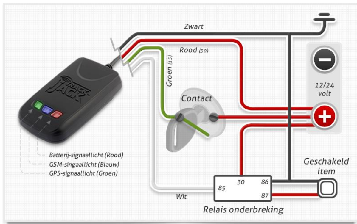
Afb. 3: aansluitschema relais
